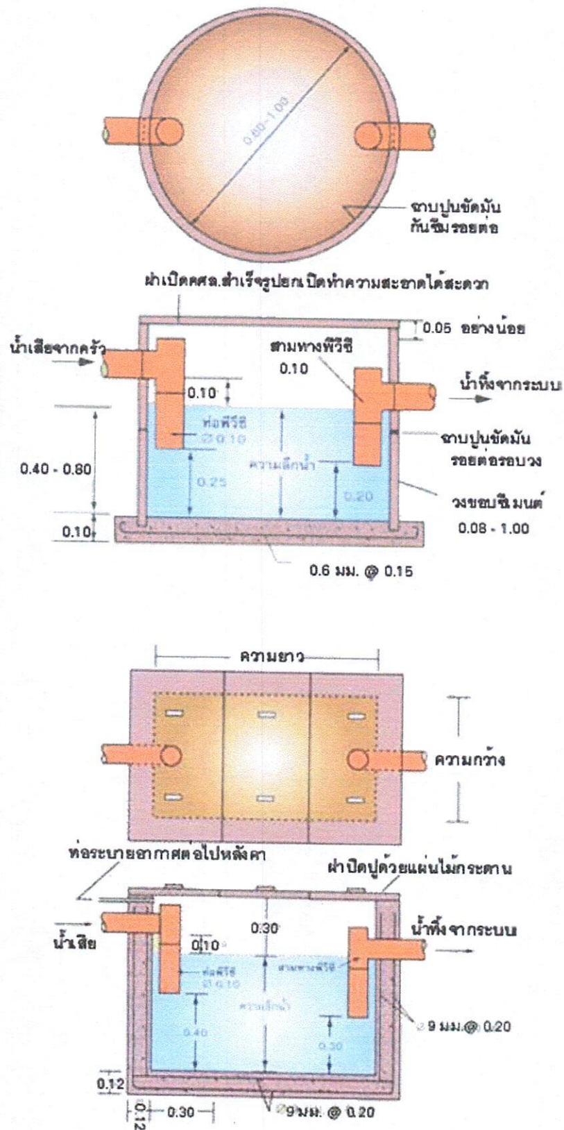
ภาพแสดงบ่อดักไขมัน
